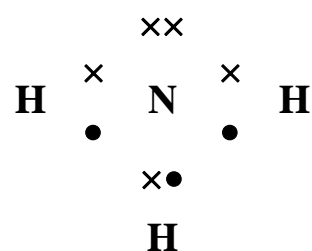
Ammonia ( NH_3 )
